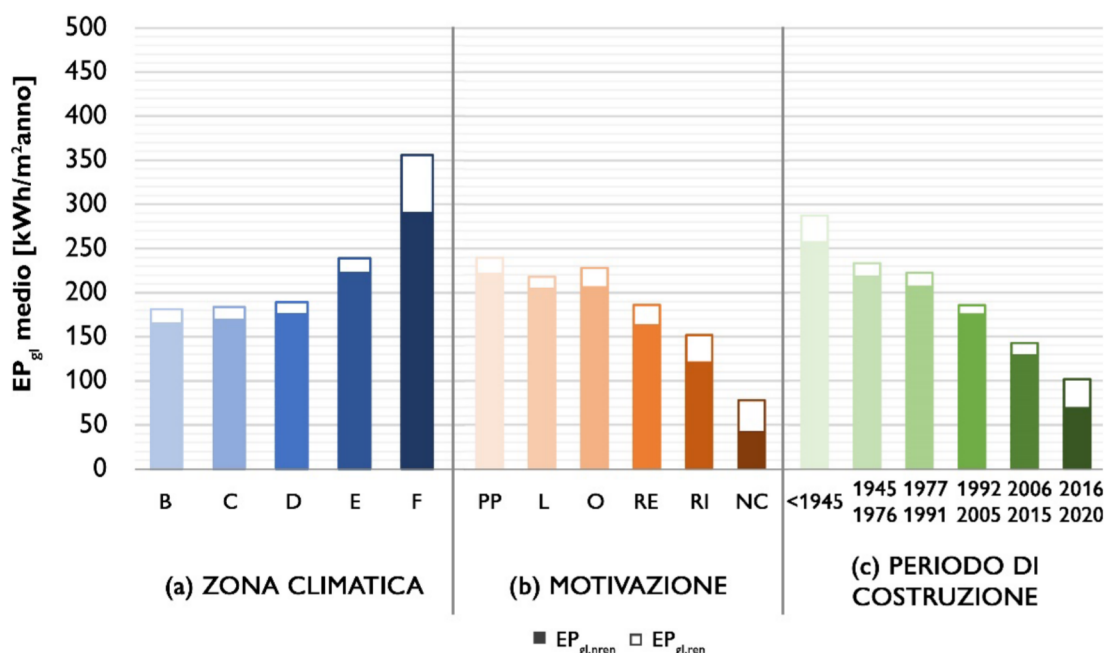
Figura 1. Distribuzione dell'EP gl medio per zona climatica (a), motivazione (b) e periodo di costruzione (c) per gli immobili residenziali. PP: passaggio di proprietà; L: locazione; A: altro; RE: riqualificazioni energetiche; RI: ristrutturazione importante; NC: nuove costruzioni (fonti: Regioni e Province Autonome e SIAPE)
