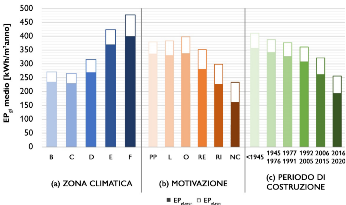
Figura 2. Distribuzione dell' EP_{gl} medio per zona climatica (a), motivazione (b) e periodo di costruzione (c) per gli immobili non residenziali. PP: passaggio di proprietà; L: locazione; A: altro; RE: riqualificazioni energetiche; RI: ristrutturazione importante; NC: nuove costruzioni (fonti: Regioni e Province Autonome e SIAPE)
