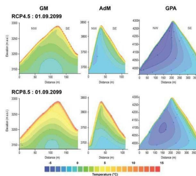
Sezioni di temperatura delle pareti rocciose per tre siti nel massiccio del Monte Bianco, secondo gli scenari RCP 4.5 e 8.5 (Aiguille des Grands Montets, Aiguille du Midi e Grand Pilier d'Angle) a fine secolo. Cambiamenti climatici nell'area del Monte Bianco e impatti sulle attività umane (Rapport Climat - Cambiamenti climatici nell'area del Monte Bianco e impatti sulle attività umane - novembre 2019). Fonte: Magnin et al., 2017, EDYTEM/CRNS
