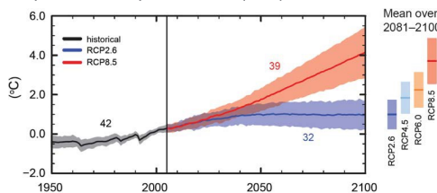
Temperatura Media Superficiale Globale (TMSG)
