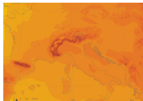
Aumento della temperatura 2021-2050
