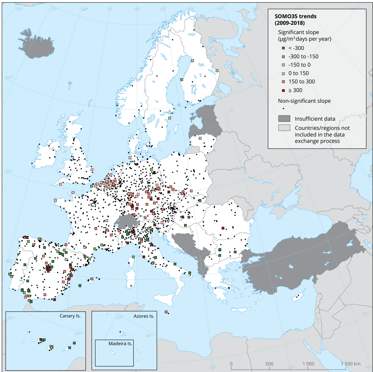
Map 5.2 SOMO35 trends (2009-2018)
