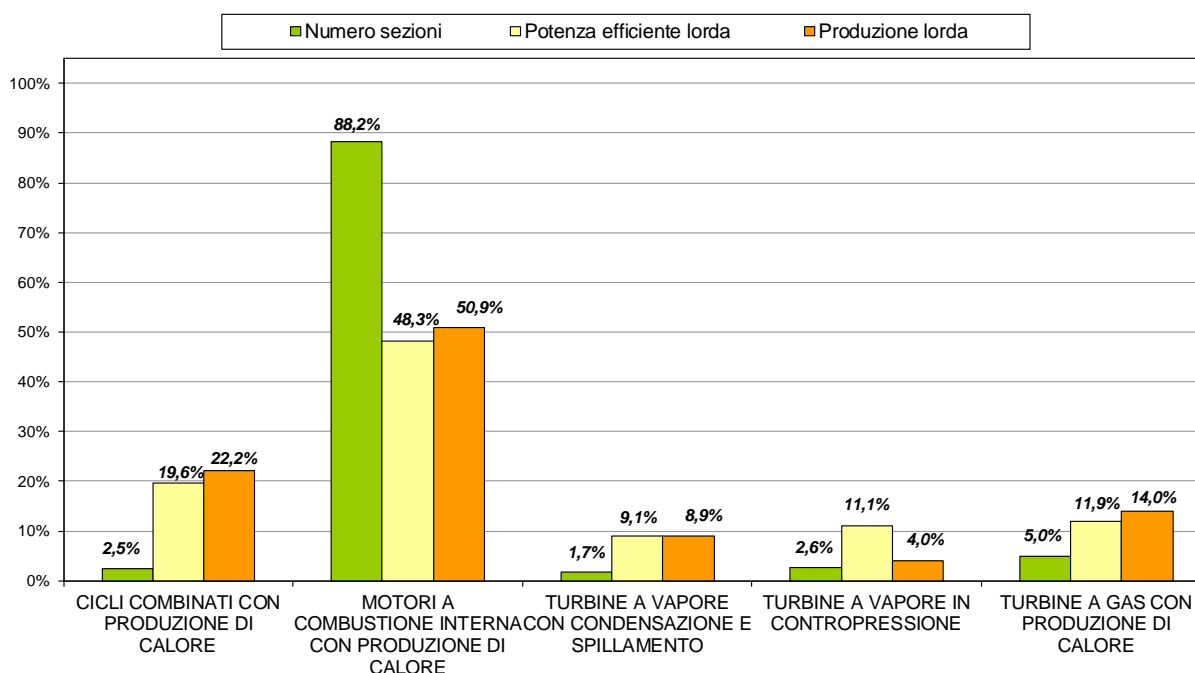
Figura 2.24: Ripartizione delle sezioni degli impianti termoelettrici tra le diverse tecnologie utilizzate per la produzione combinata di energia elettrica e calore nell'ambito della GD
