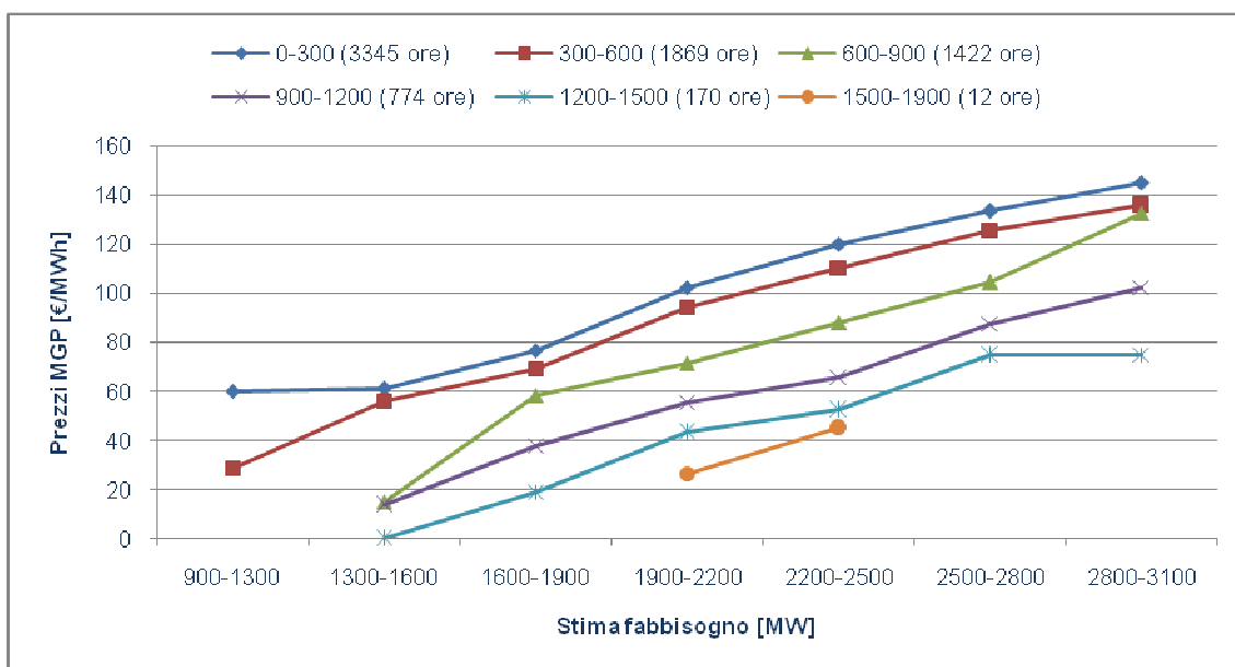
Figura 5. Andamento del prezzo medio in esito al MGP in funzione del fabbisogno e del livello di previsione di produzione eolica e fotovoltaica per la zona Sicilia (solo ore di zona Sicilia separata) - Anno 2014 (Fonte: elaborazione assoRinnovabili su dati Terna e GME)
