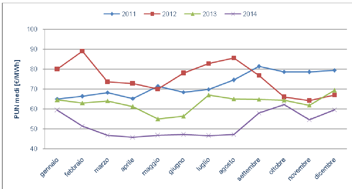
Figura 2: come si vede i valori del 2014 rappresentano il minimo storico del periodo considerato (2011 – 2014), con una particolare flessione tra marzo e agosto 2014, in cui il PUN medio è rimasto stabilmente al di sotto dei 50 €/MWh).
