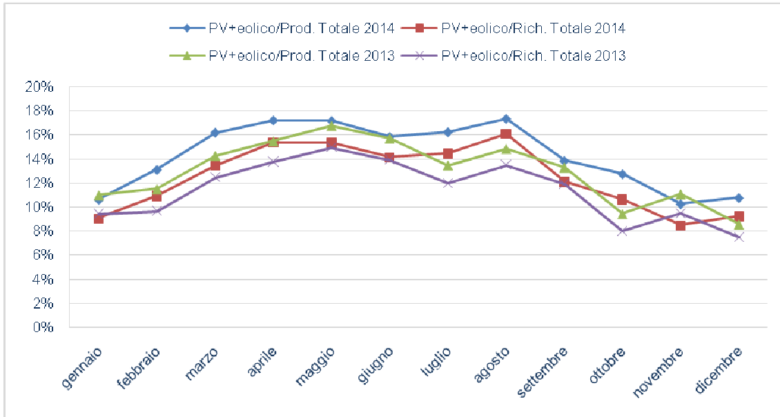
Figura 3. Andamento della produzione mensile eolica e fotovoltaica per gli anni 2013 e 2014 rispetto alla produzione e alla richiesta totali (Fonte: elaborazione assoRinnovabili su dati Terna)
