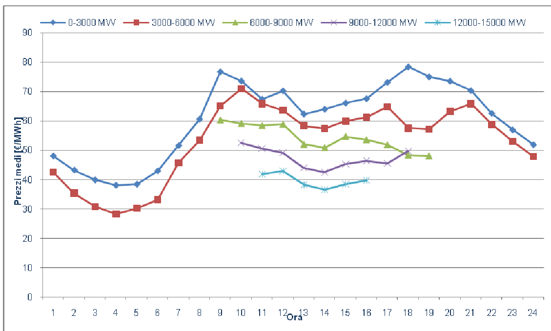
Figura 8. Andamento dei valori medi orari di PUN in funzione del livello di previsione di produzione eolica e fotovoltaica - Anno 2014 (solo giorni feriali). Fonte: elaborazione assoRinnovabili su dati Terna e GME)
