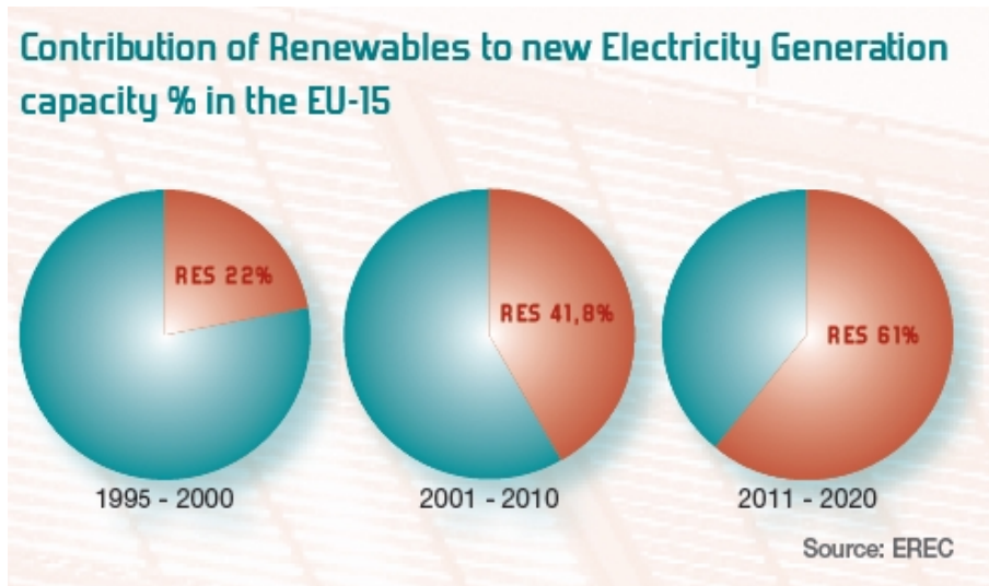
Fig. 1 Il ruolo sempre maggiore della potenza (e quindi degli investimenti) nella produzione di energia elettrica da rinnovabili in Europa
