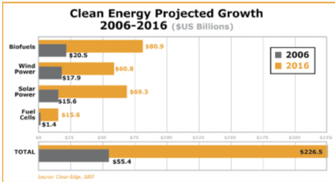
Fig.2 Il boom degli investimenti nelle fonti rinnovabili nel mondo
